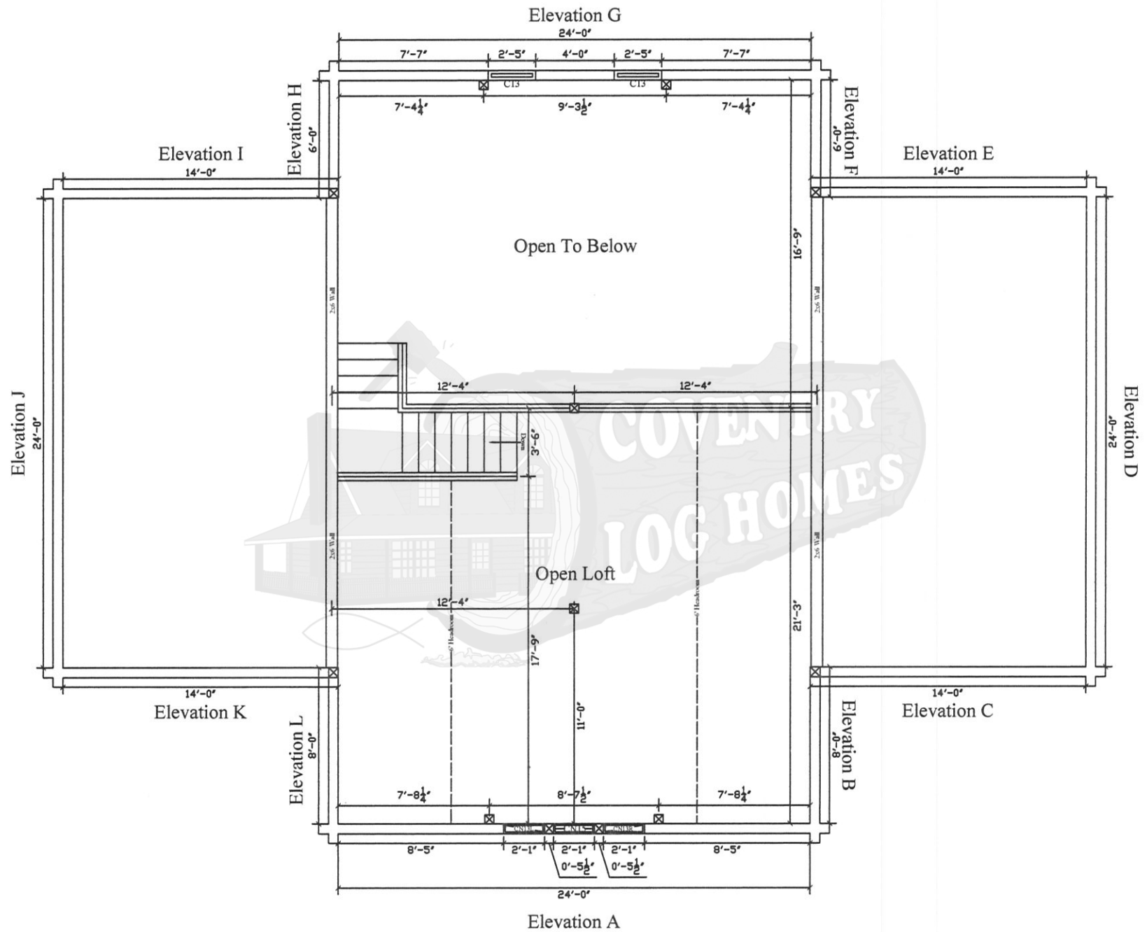
LOFT PLAN
